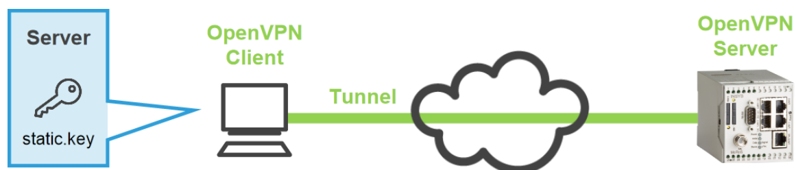
Abbildung 1: Windows-PC als OpenVPN-Client mit Authentifizierung über statischen Schlüssel
